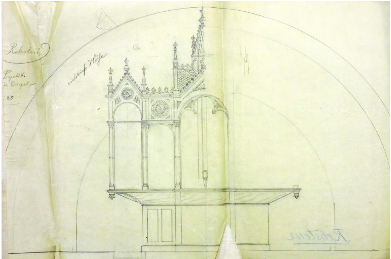
Abb. 101: Rebstein SG, katholische Pfarrkirche St. Sebastian, Zeichnung der Orgel (Archiv Orgelbau Goll, Mappe Rebstein).
