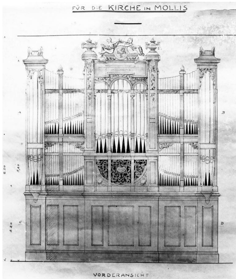
Abb. 51: Mollis GL, reformierte Kirche, der Prospektentwurf von Streiff & Schindler (Landesarchiv Glarus, Fotosammlung, Inv. Nr. 245).
