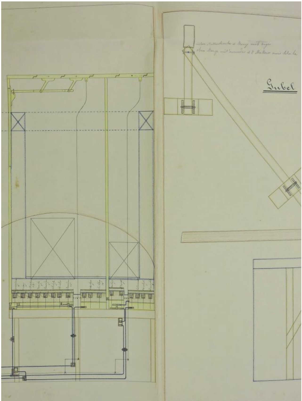
Abb. 12: Menziken ZG, katholische Kapuzinerinnenkirche Maria Hilf auf dem Gubel (Plan im Archiv Orgelbau Goll).
